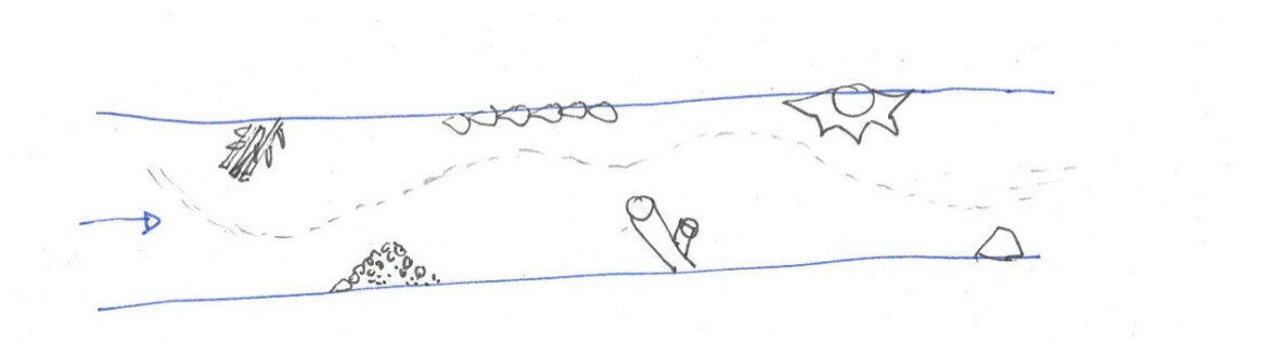
Abb. 9: Einbauweisen zur Entwicklung einer Niedrigwasserrinne
