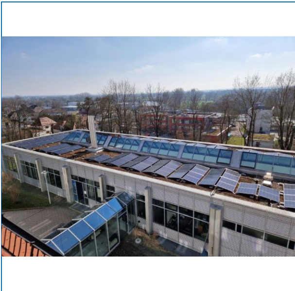
Abb. 2: Blick auf die Photovoltaik-An- lage auf dem Dach des La- borgebäudes.
